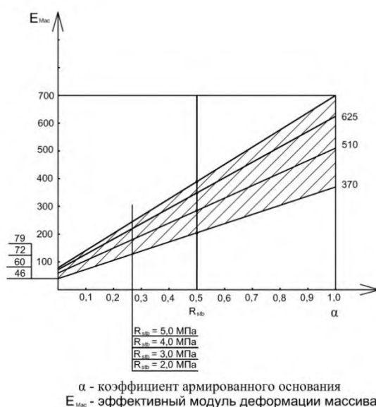
Рисунок Ф.1 – График зависимости эффективного модуля деформации армированного ГЦЭ массива от коэффициента армирования при прочности грунтоцемента – 2, 3, 4, 5 МПа для песков (коэффициент армирования – отношение в долях единиц объема ГЦЭ к объему закреплённого грунта)
