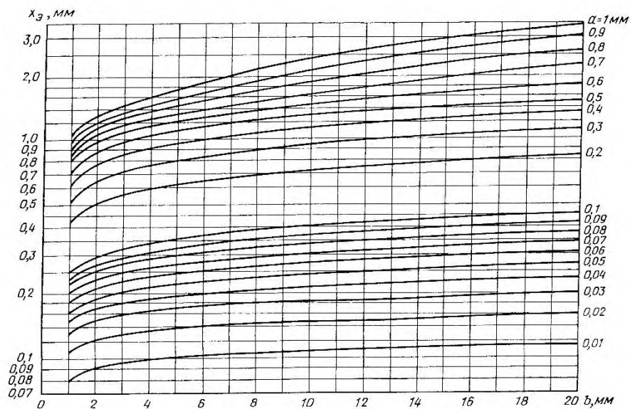
Рисунок Б.1 — Номограмма для определения эквивалентного размера протяженных объектов различения при расстояниях от глаза до объекта до 500 мм
