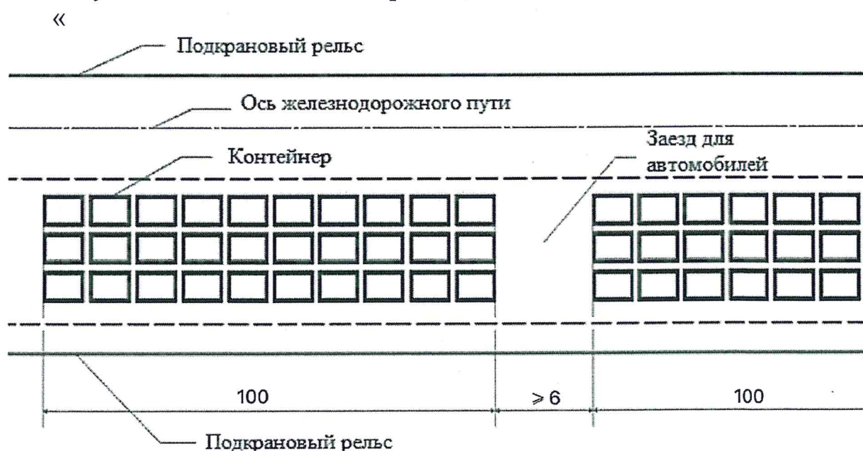
Рисунок 4 – Схема поперечного заезда автомобилей
