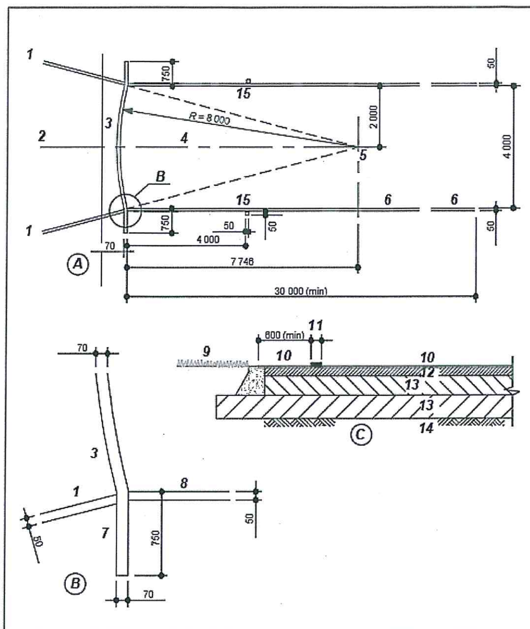
А – общая схема; В – подробный план; С – продольное сечение; 1 – разметка сектора для метания; 2 – зона приземления; 3 – ограничительная дуга; 4 – усиленный участок дорожки для разбега; 5 – центр – точка пересечения схемы; 6 – дорожка для разбега; 7 – разметка краев дуги, выходящих за дорожку; 8 – разметка боковых границ дорожки; 9 – травяное покрытие; 10 – синтетическое покрытие; 11 – разметка дуги; 12 – асфальтобетон; 13 – гравиевая подложка; 14 – грунтовое основание; 15 – белые отметки 0,05×0,05 м
