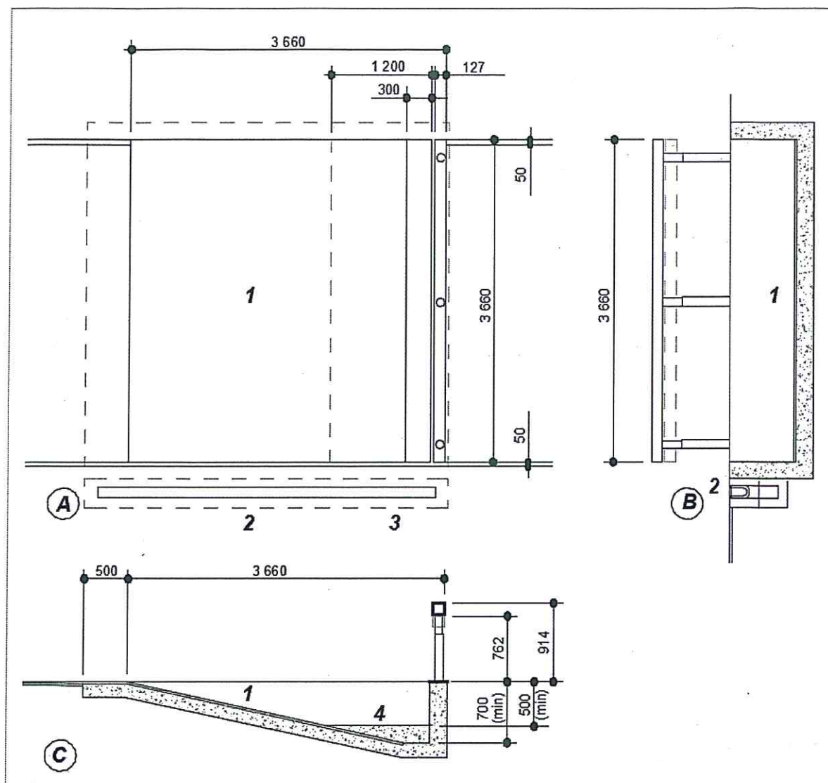
A – план; B – поперечное сечение; C – продольное сечение; 1 – синтетическое покрытие, 25 мм; 2 – дренажный водосток; 3 – закрывающийся водосток; 4 – бетонный каркас для стационарных ям с водой (необязательный компонент)
