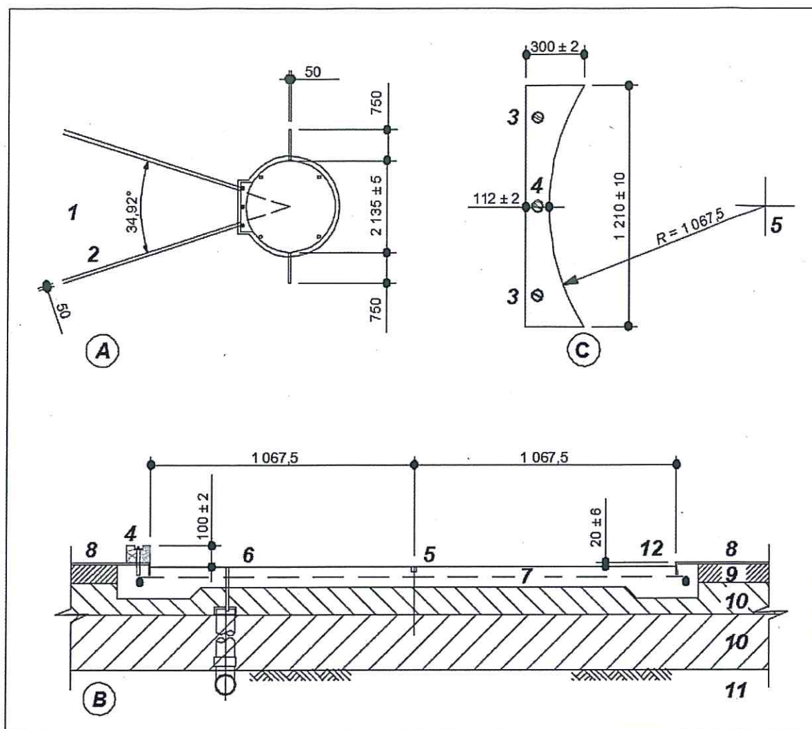
А – общая схема; В – подробный план в сечении; С – сегмент; 1 – сектор приземления; 2 – разметка сектора приземления; 3 – крепежная вставка; 4 – сегмент; 5 – отверстие в центре круга диаметром 4 мм; 6 – дренажная труба; 7 – армированное бетонное основание; 8 – синтетическое покрытие; 9 – асфальтобетон; 10 – гравиевая подложка; 11 – грунтовое основание; 12 – металлический обод
