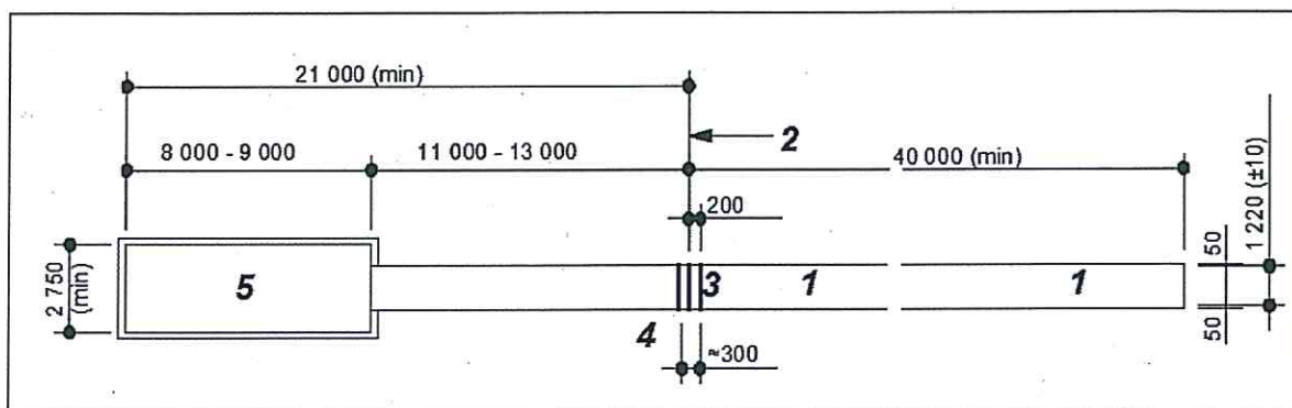
Рисунок Е.11 – Минимальное расстояние между параллельно расположенными секторами для прыжков в длину и тройного прыжка
