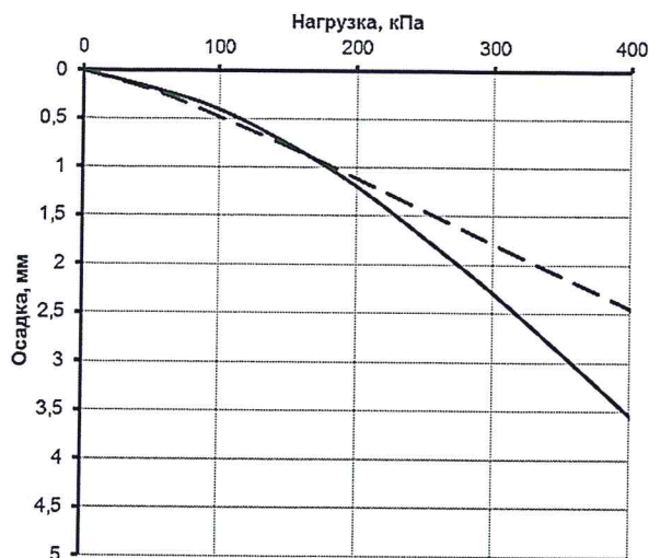
а) Штамповые испытания – удовлетворительное описание
