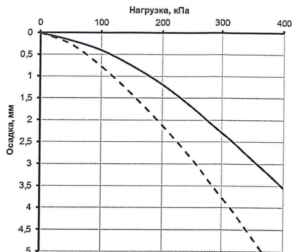
б) Штамповые испытания – неудовлетворительное описание
