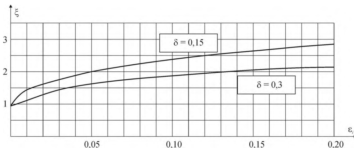
Рисунок 11.1 – Коэффициенты динамичности
