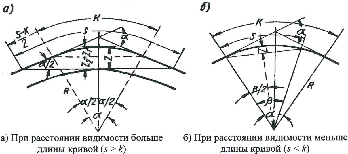
Рисунок Г.1– Препятствия для видимости в плане
