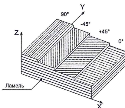
Рисунок 12.1 – Пример строения ламината конструктивных элементов
