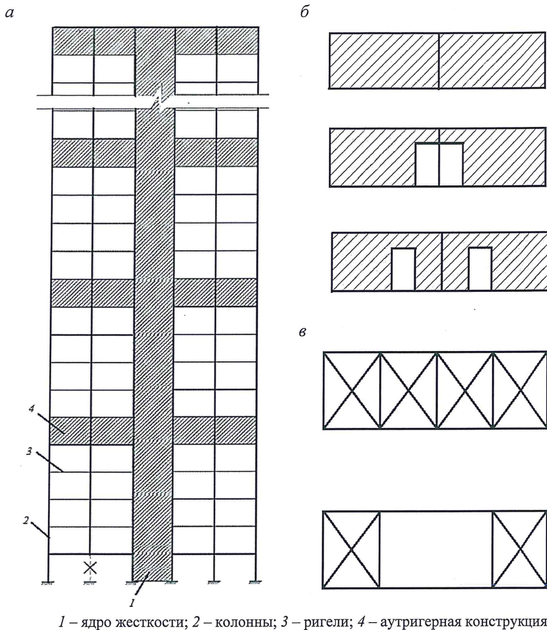
Рисунок 9.2 – Схема расположения аутригерных конструкций (а) и типы этих конструкций сплошного (б) или сквозного (в) сечения
