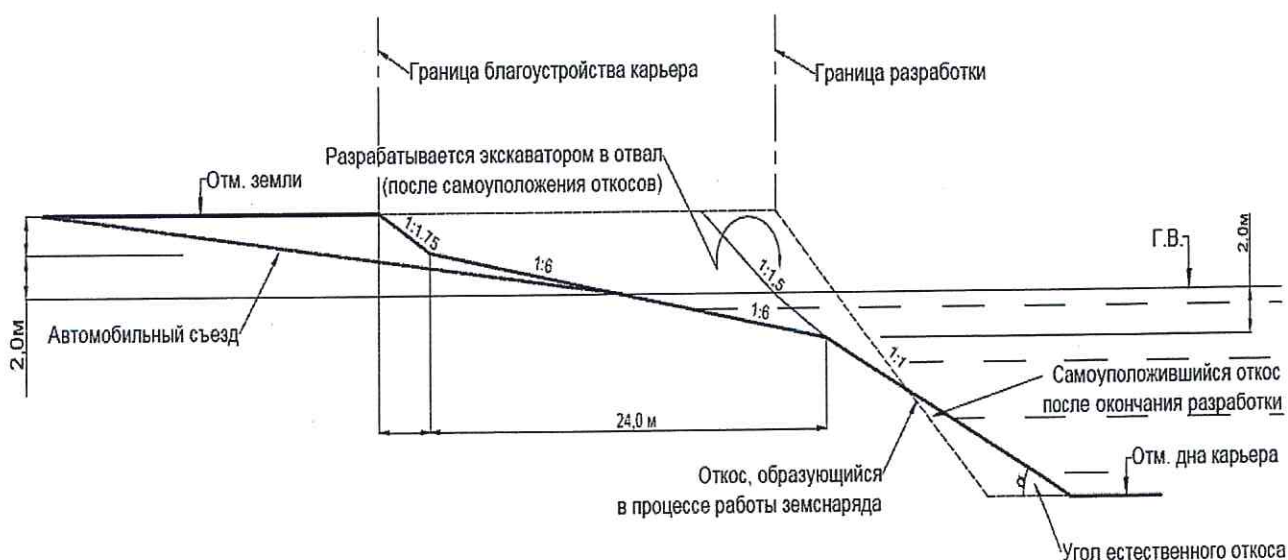
Рисунок К.3 – Водоем для технических нужд (вариант А)
