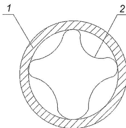
1 – муфта; 2 – уплотнитель
