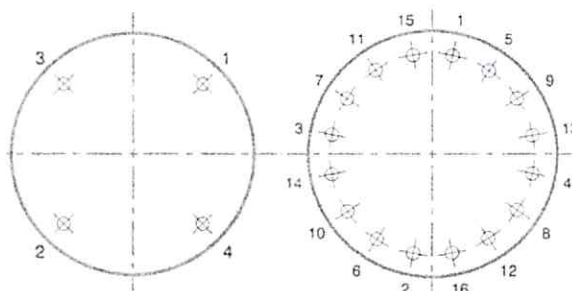
Рисунок 14 – Схема последовательности затяжки болтов
