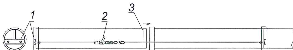
Рисунок 8 – Наружная стыковка труб с помощью ручной (рычажной) тали
