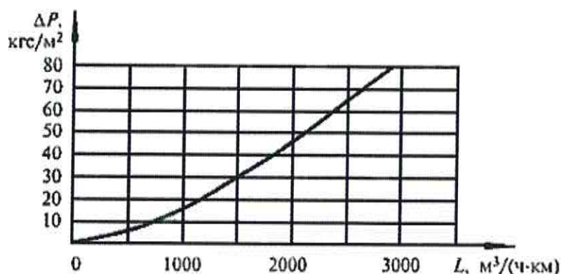
Рисунок В.1 – График нормируемой утечки воздуха в испытываемом отсеке
