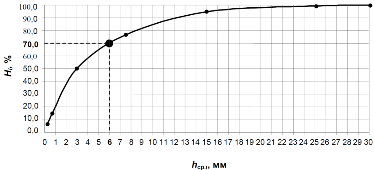
Рисунок И.1 Зависимость принимаемого на очистку суммарного за год слоя жидких осадков (%) от величины максимального суточного слоя дождя (мм), принимаемого на очистку в полном объёме, для г. Санкт-Петербург (по метеостанции Ленинград, ИЦП)
