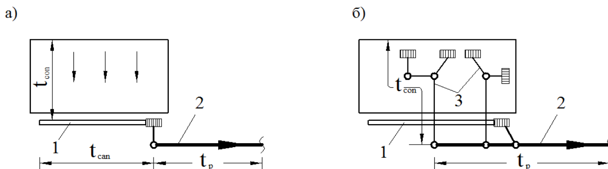
Рисунок 1 Схемы к определению продолжительности протекания дождевых вод t_r
