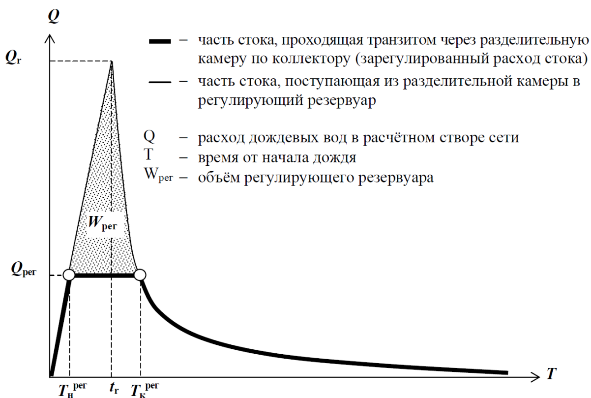
Рисунок Е.1 Гидрограф дождевого стока в сети дождевой канализации с разделительной камерой (ливнесбросом) и регулирующим резервуаром
