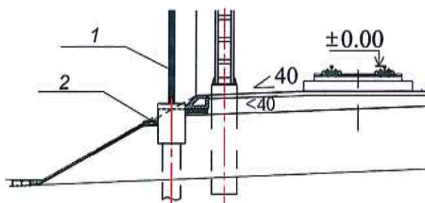
Рисунок 8.15 – Реализация поперечного водоотвода при свайном фундаменте с высоким ростверком
