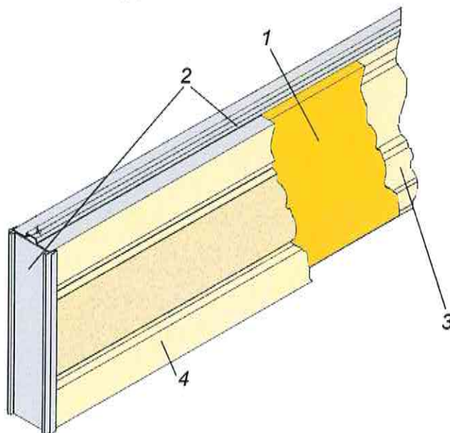
1 – звукопоглощающий материал; 2 – звукоизолирующий каркас; 3 – звукопроницаемая крышка; 4 – звукоизолирующая крышка
