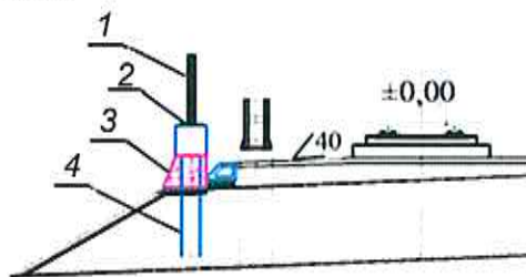
Рисунок 8.15 – Реализация поперечного водоотвода при свайном фундаменте с высоким ростверком
