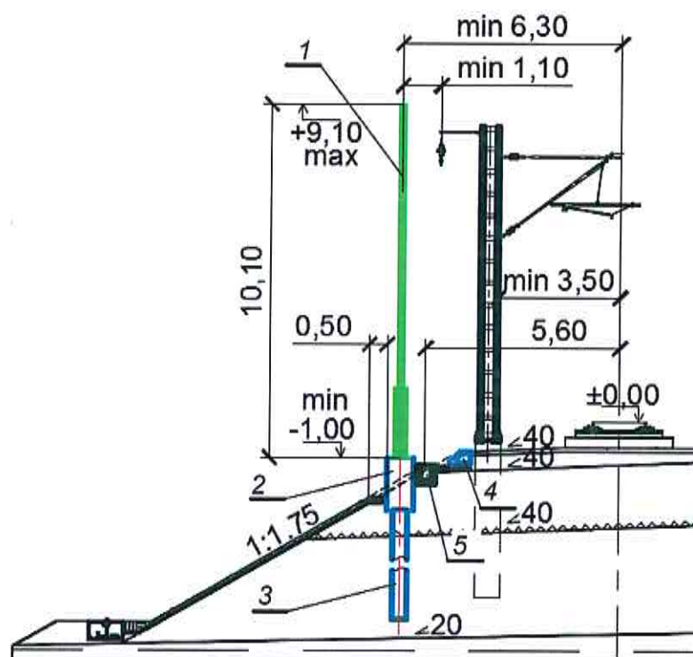
Рисунок 8.21 – Пример установки шумозащитного экрана на основной площадке земляного полотна за пределами верхнего строения пути
