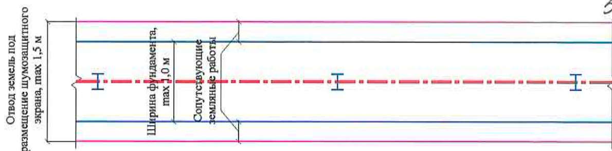
Рисунок 8.3 – Схема определения габаритных размеров отвода земель под шумозащитный экран
