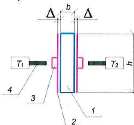
1 – испытываемая панель; 2 – распределительный лист; 3 – площадка для штока толкателя; 4 – шток толкателя; b – толщина панели; h – высота панели; T_1 , T_2 – толкатели; \Delta – величина опытного прогиба
