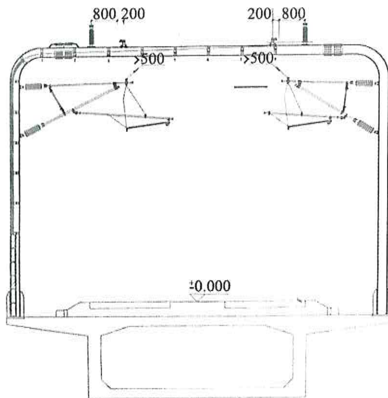
Рисунок 8.10 – Выполнение тоннельных галерей и совмещение конструкций
