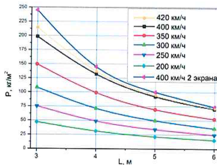
Рисунок 8.5 – График учета аэродинамической нагрузки для прямого шумозащитного экрана
