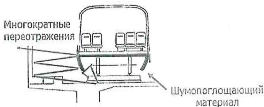
Рисунок 7.1 – Схема облицовки шумопоглощающим материалом тележки поезда
