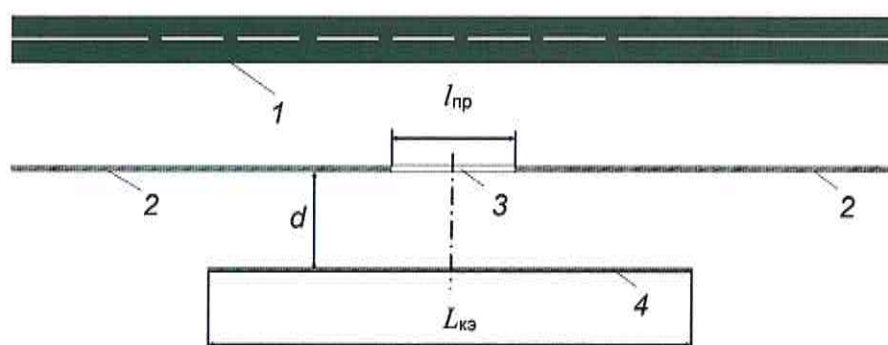
1 — железнодорожный путь; 2 — ШЭ; 3 — технологический проход (разрыв); 4 — контрэкран; d — расстояние до контрэкрана; L_{кэ} — длина контрэкрана; l_{пр} — длина прохода
