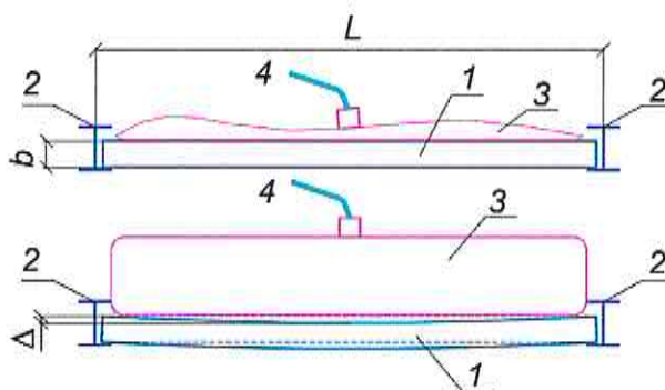
1 — испытываемая панель; 2 — элемент крепления; 3 — резервуар с водой; 4 — вода
