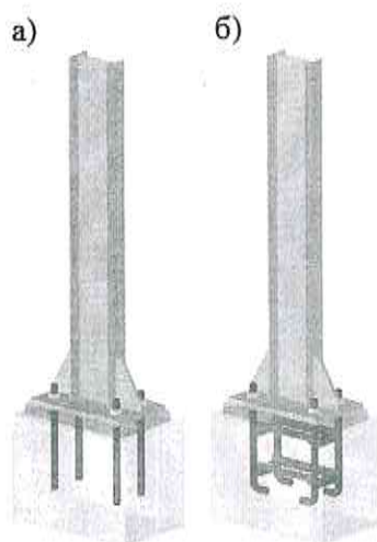
а – глухие несъемные болты, устанавливаемые с применением химических клеевых составов; б – глухие несъемные болты, устанавливаемые до бетонирования, объединенные в пространственную группу
