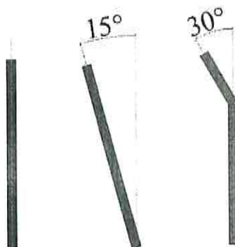
Рисунок 8.6 – Формы шумозащитных экранов, для которых допускается не учитывать снеговые нагрузки
