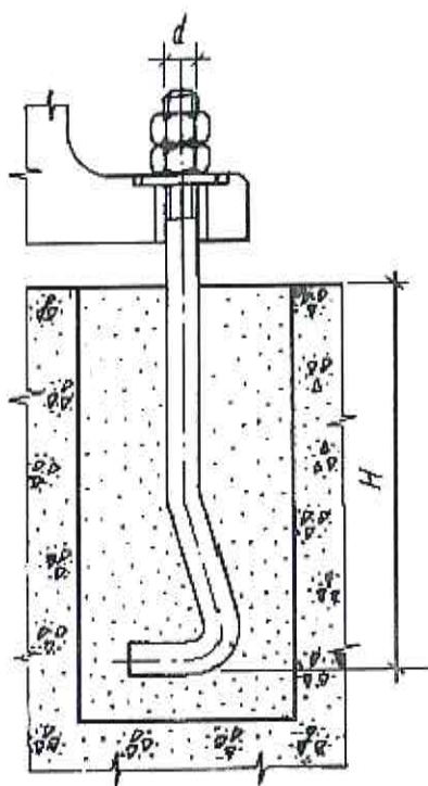
Рисунок 8.20 – Замененный фундаментный болт
