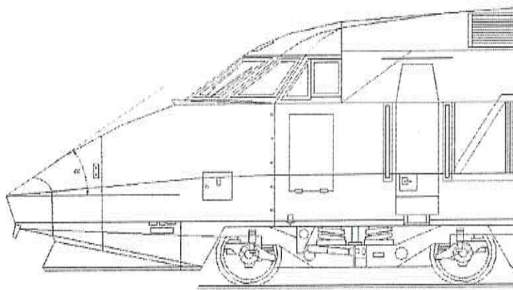
Рисунок 6.1 – Определение внутреннего угла \alpha лобовой части поезда
