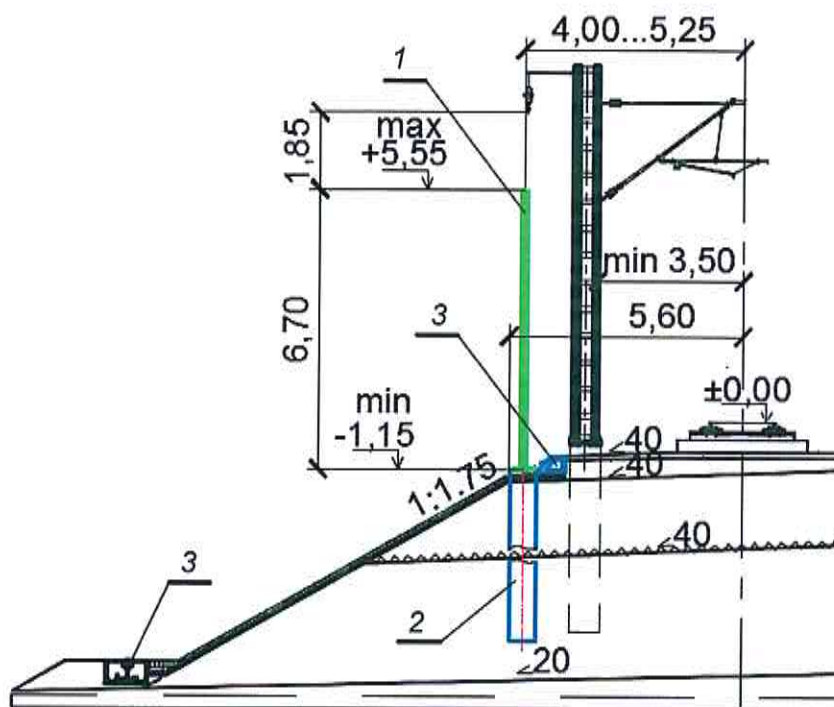
Рисунок 8.21 – Пример установки шумозащитного экрана на основной площадке земляного полотна за пределами верхнего строения пути
