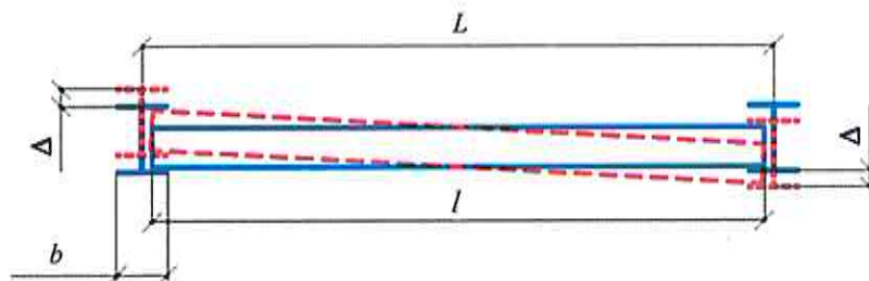
Рисунок 8.8 – Схема расчета предельных перемещений свободных концов несущих элементов
