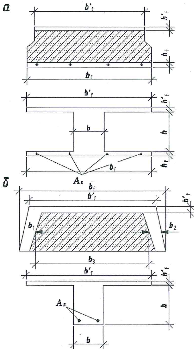
а – плита перекрытия трехслойная; б – плита перекрытия с боковыми несущими гранями
