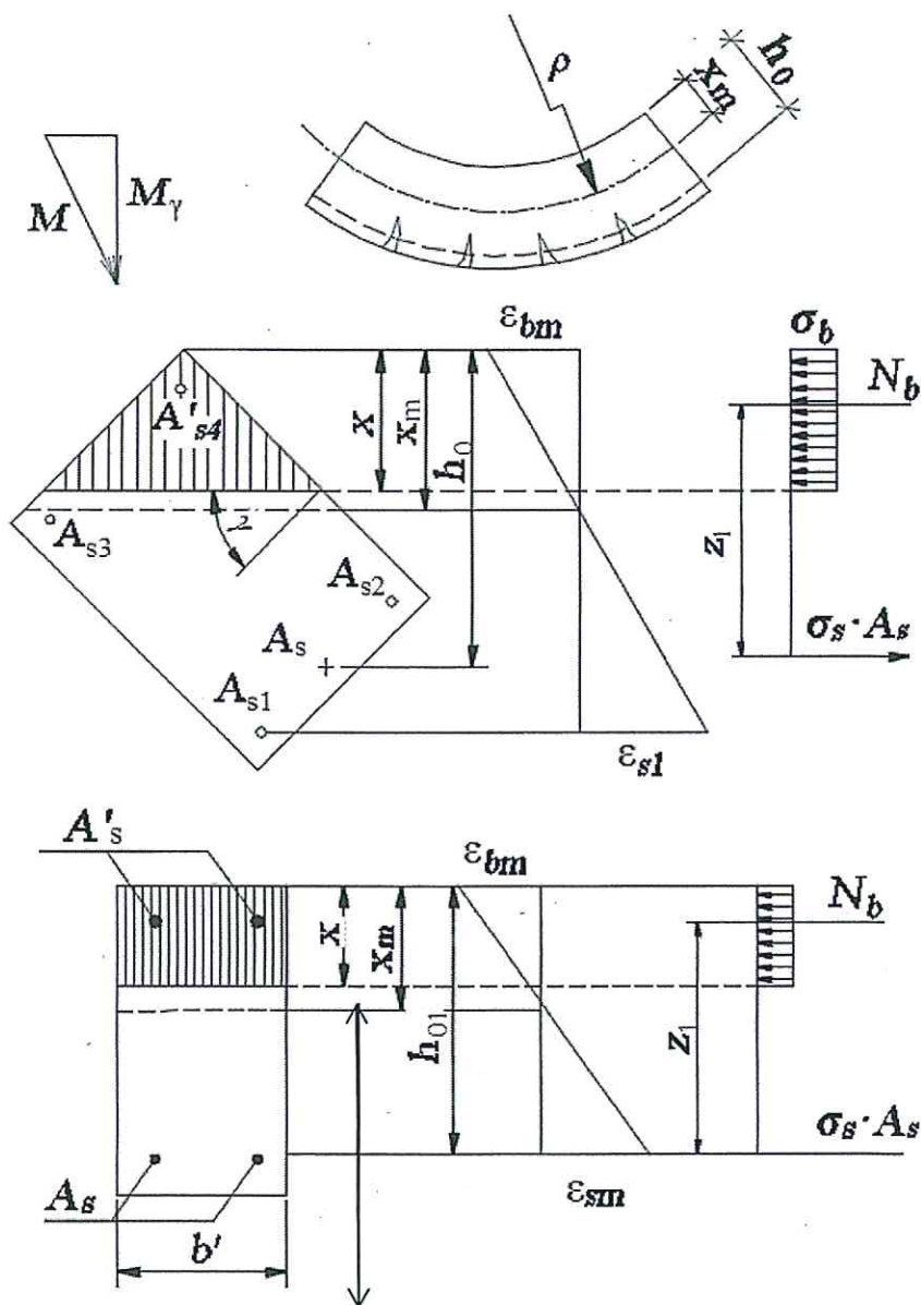
Рисунок Д.1 – Напряженно-деформированное состояние элементов при косом и плоском изгибе
