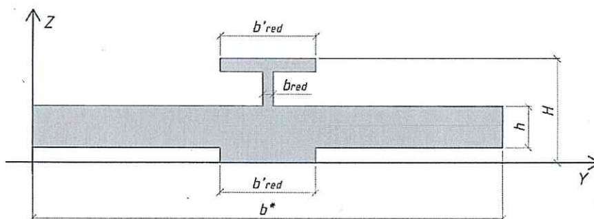
Рисунок 7.21 – Приведенное поперечное сечение ограждающих конструкций
