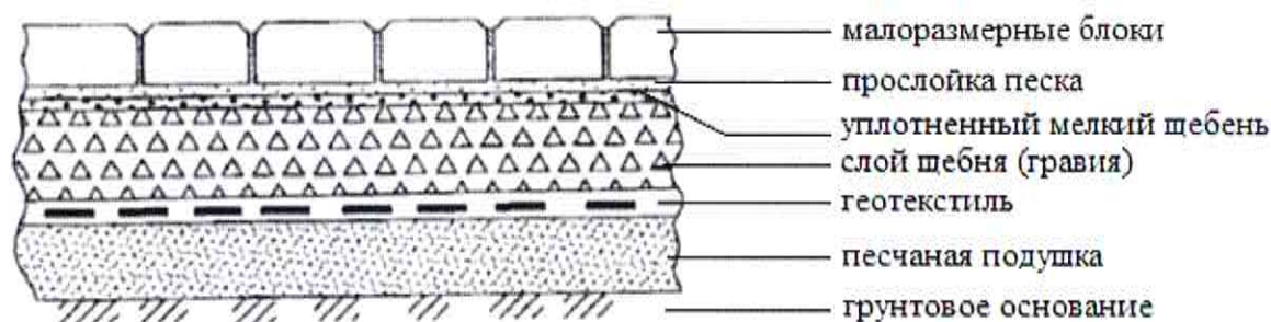
Рисунок 6 – Блочные покрытия
